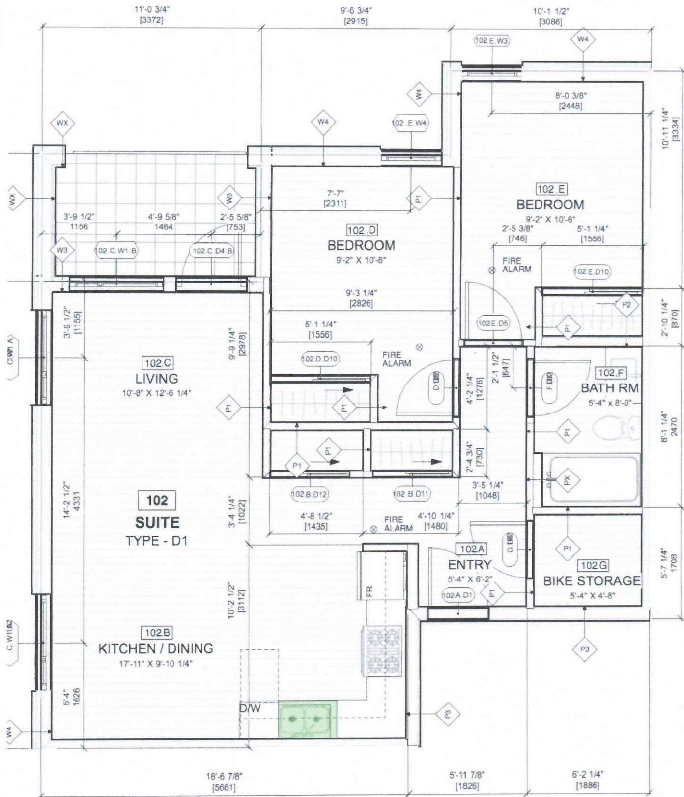
Unit D1 2 Bed + 1 Bath AVG. GFA = 72.23 sq. m.
